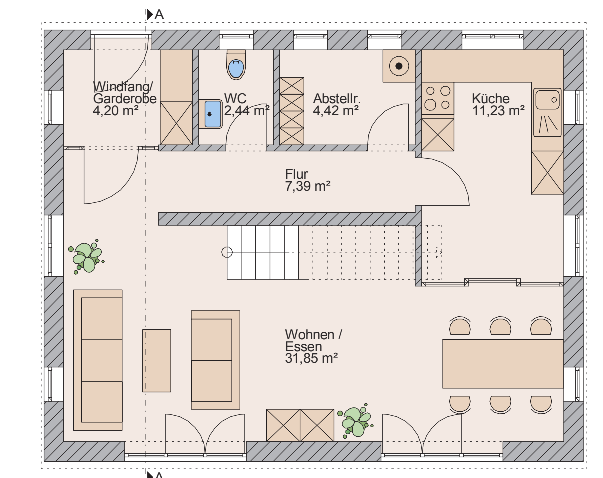
Variante 2 Grundriss Erdgeschoss
