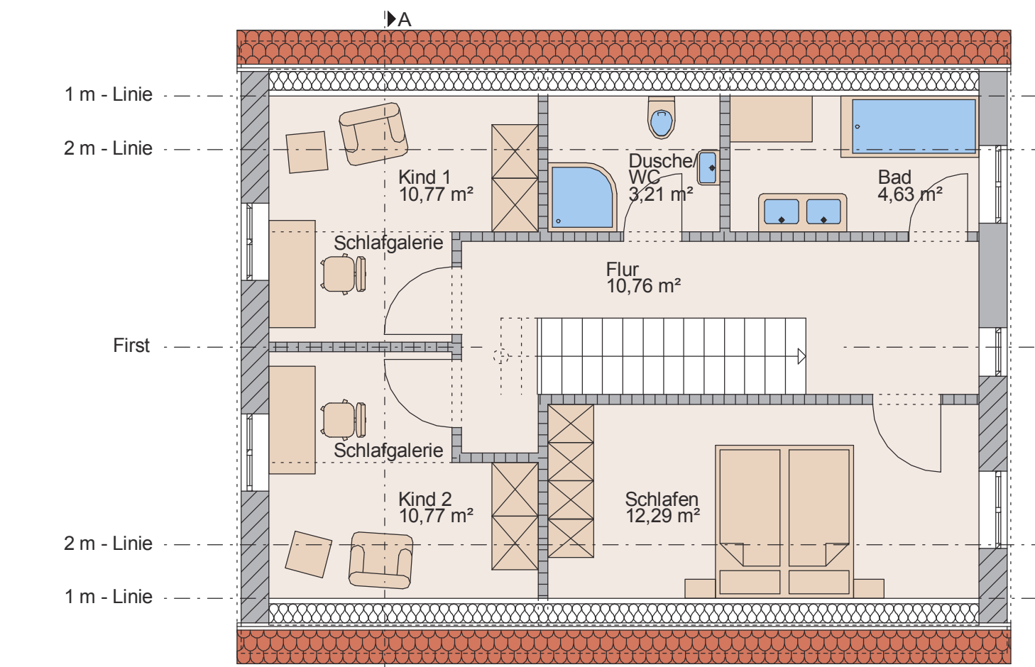
Variante 2 Grundriss Dachgeschoss
